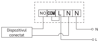
Schema de conectare a cazanului
