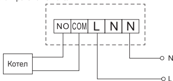
Схема на свързване на котел
