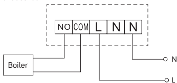
Boileri ühendusskeem
