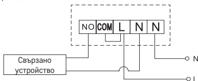
Схема на свързване на разширителен шибър/електрическо задвижване
