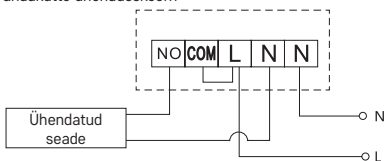
Põrandakütte ühendusskeem
