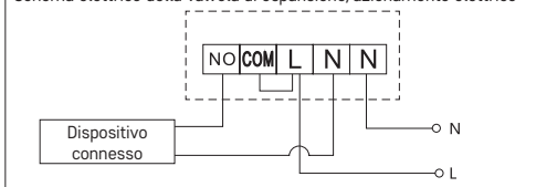
Schema elettrico della valvola di espansione/azionamento elettrico
