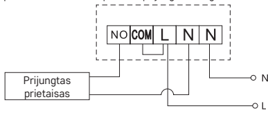
Išsiplėtimo vožtuvo / el. pavaros prijungimo diagrama
