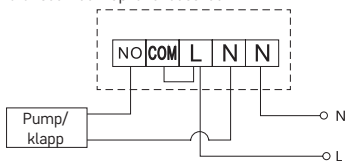
Pumba/motoriseeritud klapi ühendusskeem
